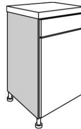
Meubles bas H.770 / 350 L.630
