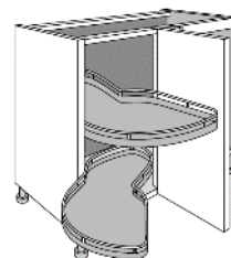
Bas angle 1 porte battante + plateaux LeMans L.1000
