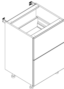
Bas 2 casseroiliers inégaux L.400/600/800/1000
