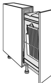
Bas 1 porte extractible Espace pain L.150
