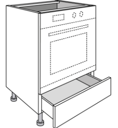
Bas four + 1 tiroir L.600
