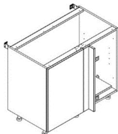
Bas angle 1 porte battante L.500 L.1000
