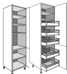
L.40- 60 Réserve 1 porte + 6 tablettes ou 5 coulissants< à l'anglaise
