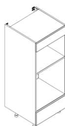
Four + MO 1 tiroir Bandeau recoupable
