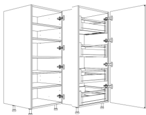
Réserve 1 porte + 4 tablettes ou 4 coulissants à l'anglaise
