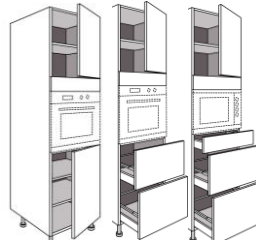
L.60 Four 2 portes + 2 tablettes ou 2 coul. + 1 P + 1 tabl. Ou 3 coul. + 1 P + 1 tabl Bandeau recoupable
