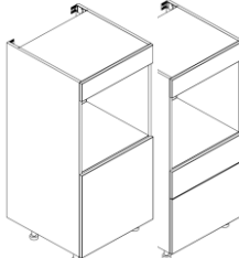
Four 1 porte + tablette Ou 2 coulissants Bandeau recoupable
